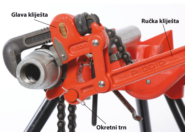
Slika 6B - Učvršćivanje ručice na držač lanca
