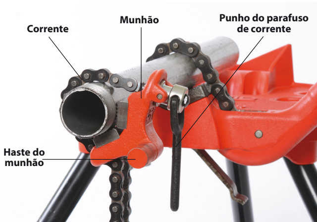
Figura 6A - Montar o munhão de alavancagem combinada no tubo
