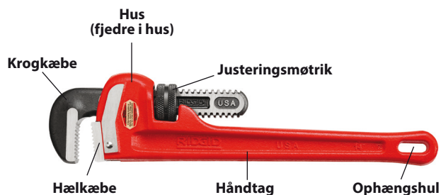
Figur 2 – Tangkomponenter
