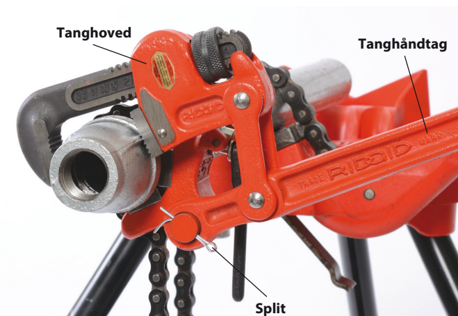
Figur 6B – Fastgørelse af håndtag på holder
