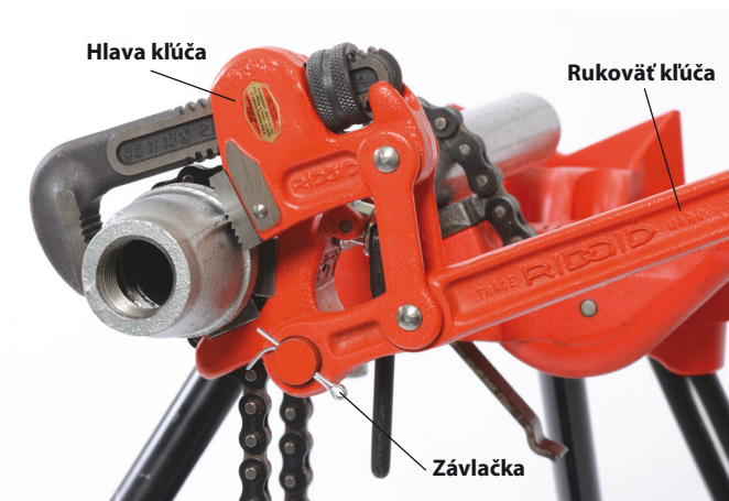
Obrázok 6B – Zaistenie rukoväti k čapu
