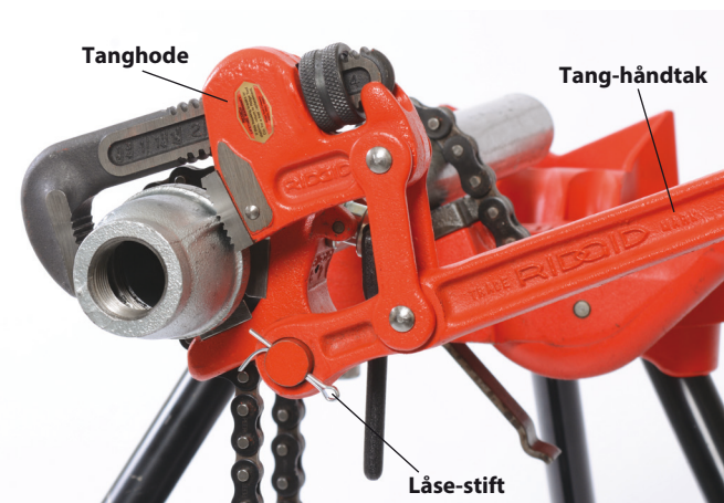
Figur 6B – Feste håndtaket til kingbolten
