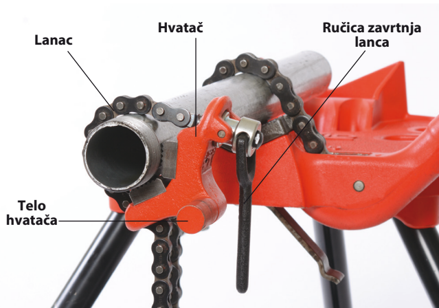
Slika 6A – Montaža hvatača francuskog ključa sa višestrukim polugom, na cev
