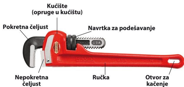
Slika 2 – Delovi ključa
