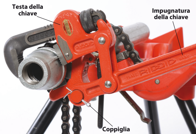
Figura 6B – Fissaggio dell'impugnatura al perno di regolazione
