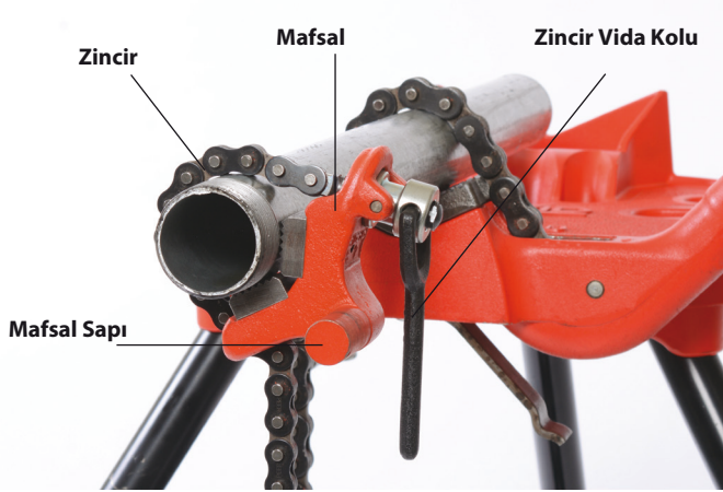
Şekil 6A - Boru Üzerindeki Bileşik Kaldıraç Anahtarı Mafsalı
