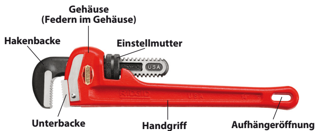
Abbildung 2 – Teile der Rohrзange
