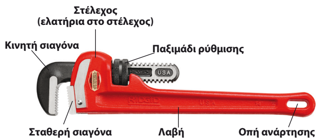
Εικόνα 2 – Εξαρτήματα σωληνοκάβουρων
