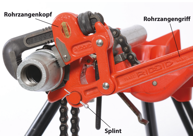
Abbildung 6B – Sichern des Griffs am Zapfen
