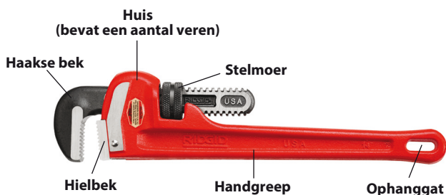
Figuur 2 – Onderdelen van de pijptang
