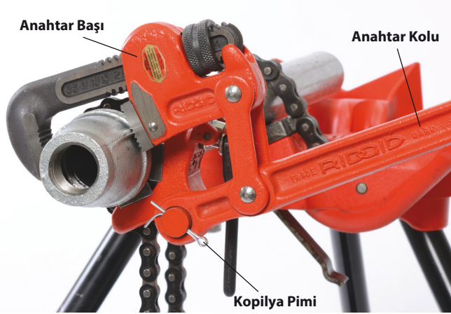
Şekil 6B - Mafsal Tutma Kolu
