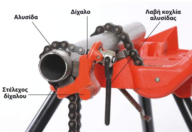
Εικόνα 6Α – Τοποθέτηση δίχαλου σύνθετου σωληνοκάβουρα σε σωλήνα
